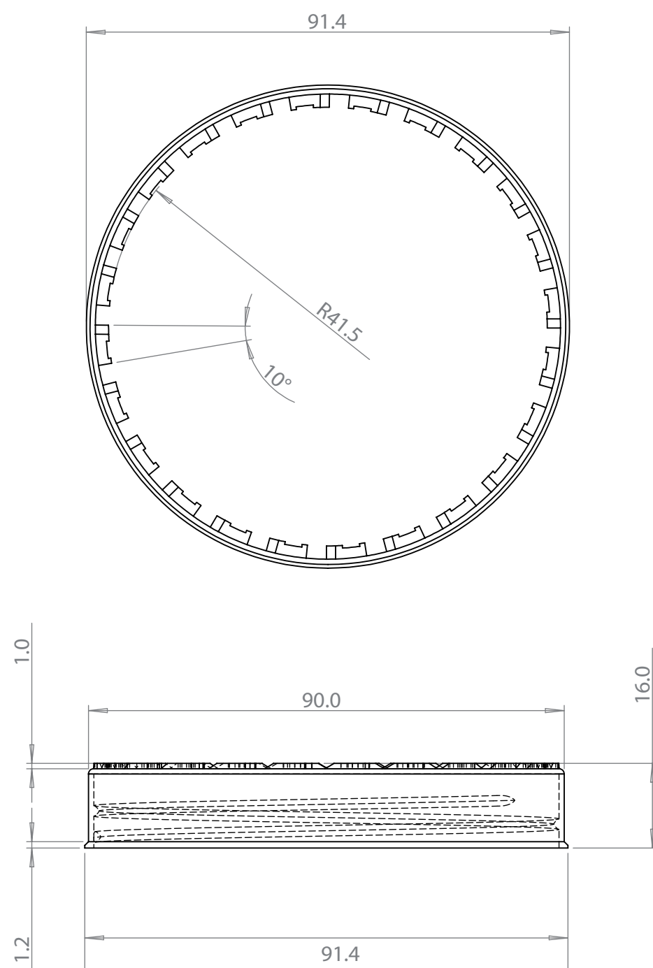
inner lid
