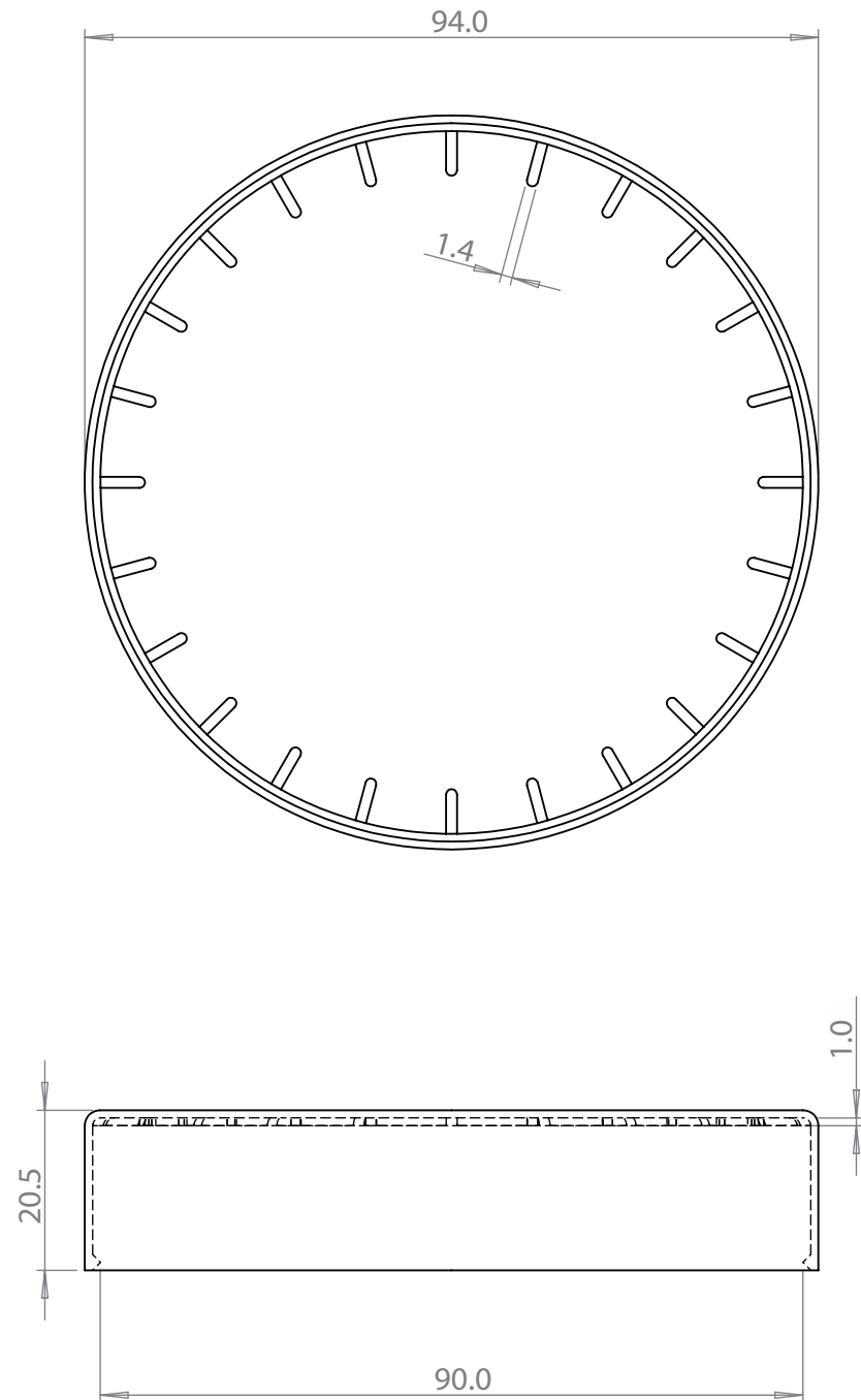
out lid
